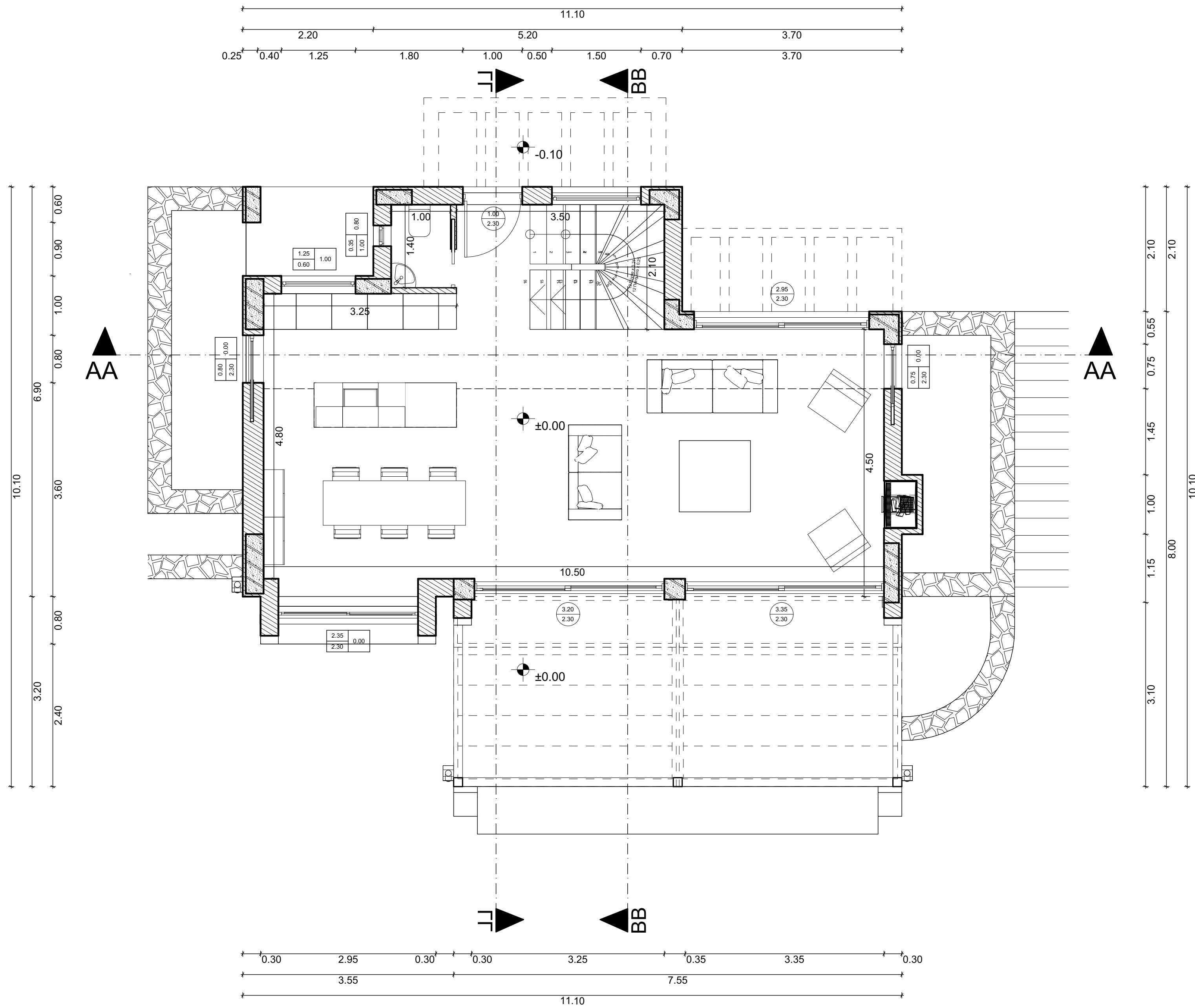
ΚΑΤΟΨΗ ΙΣΟΓΕΙΟΥ
