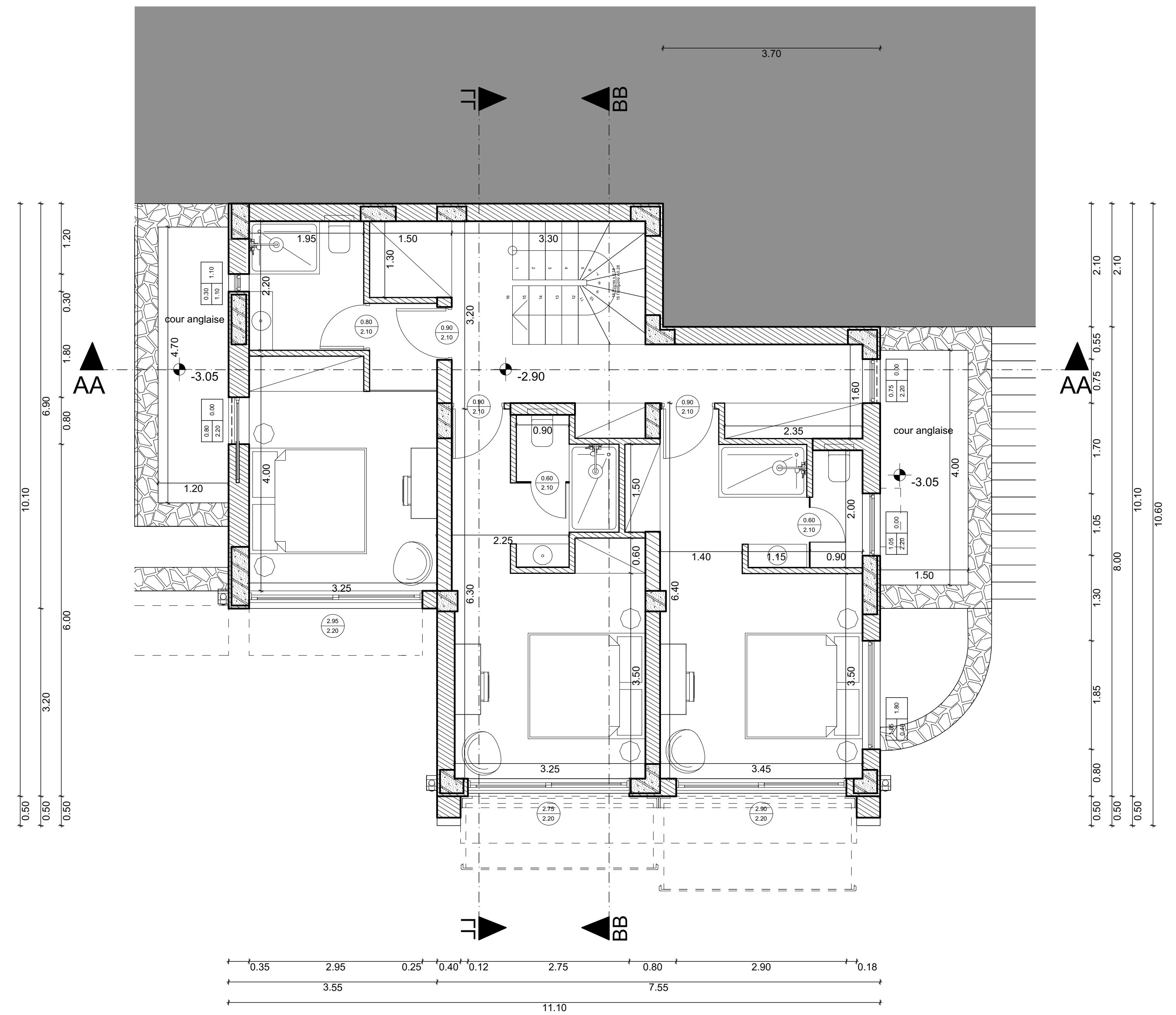
ΚΑΤΟΨΗ ΥΠΟΓΕΙΟΥ
