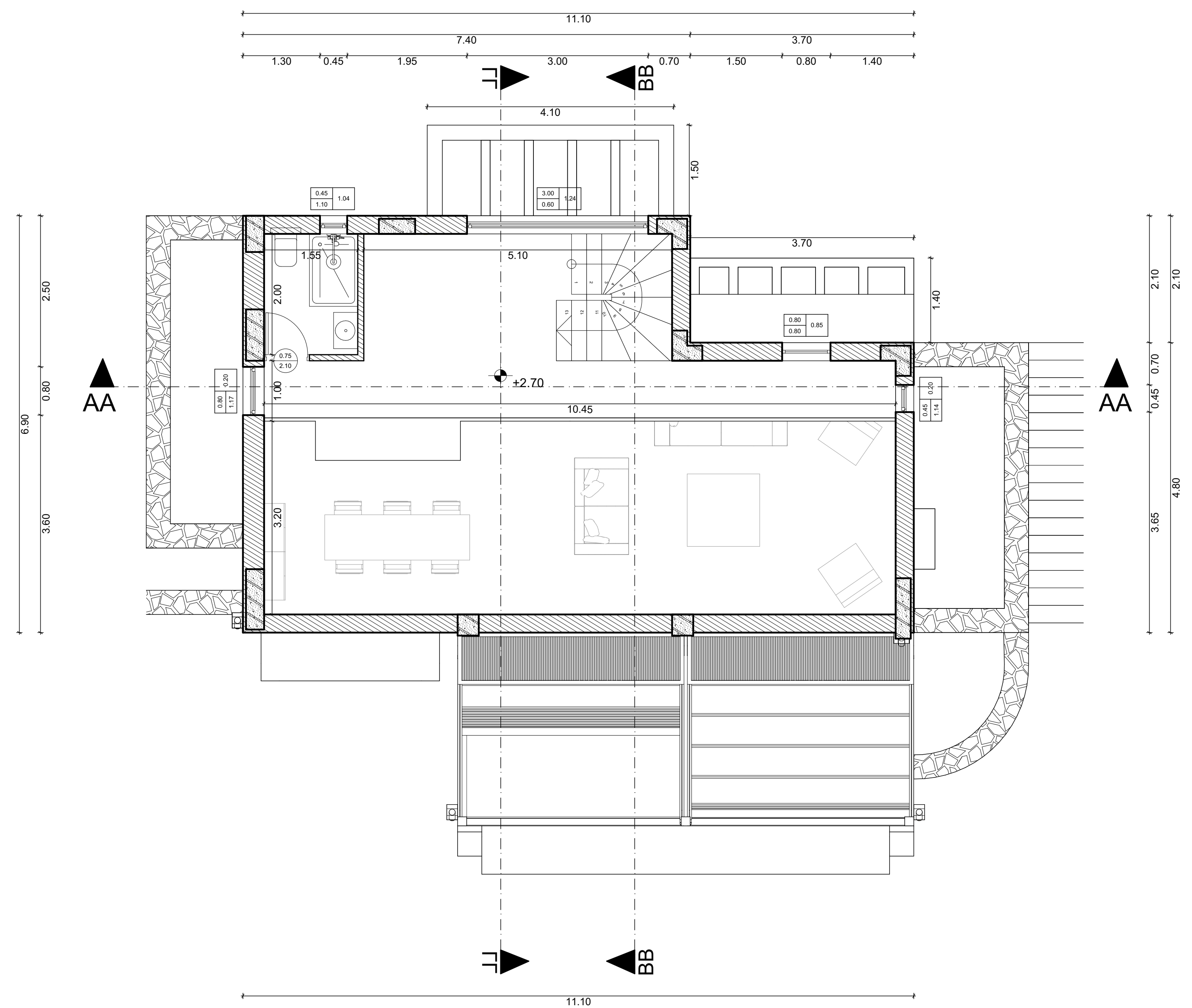
ΚΑΤΟΨΗ ΠΑΤΑΡΙΟΥ
