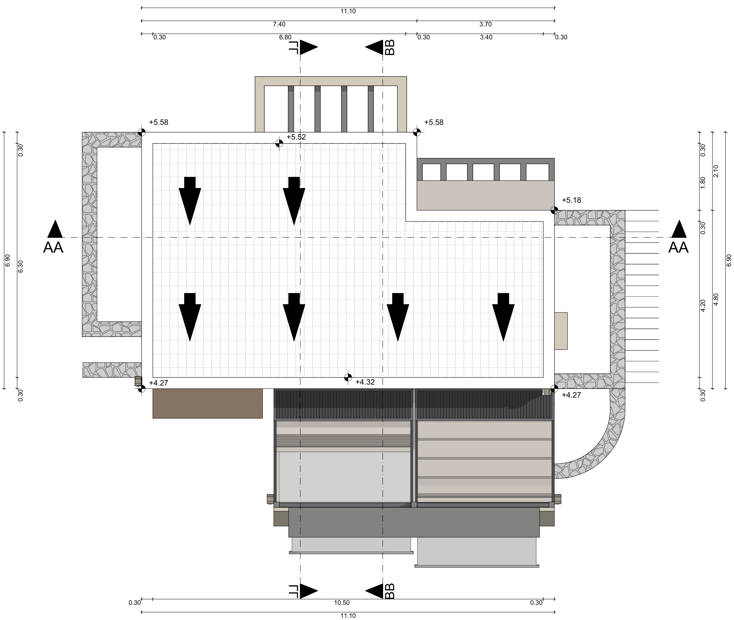
ΚΑΤΟΨΗ ΣΤΕΓΗΣ
