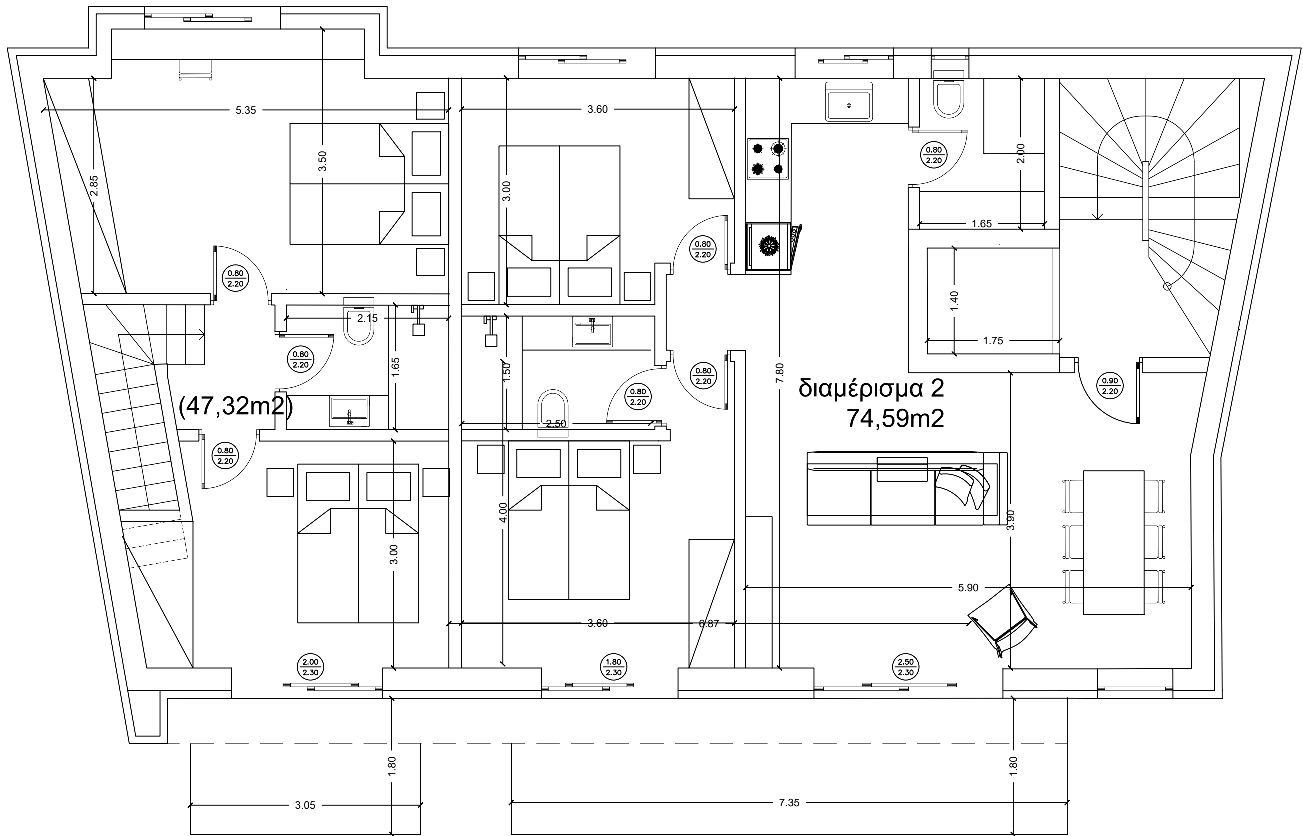
ΚΑΤΟΨΗ ΙΣΟΓΕΙΟΥ Β'
